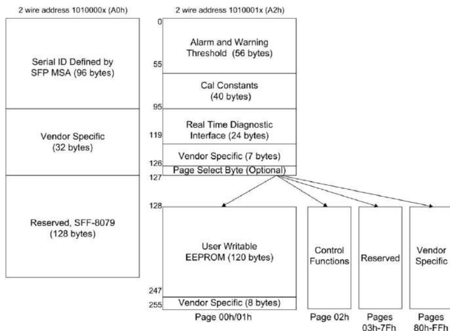
Figure4: Memory map
