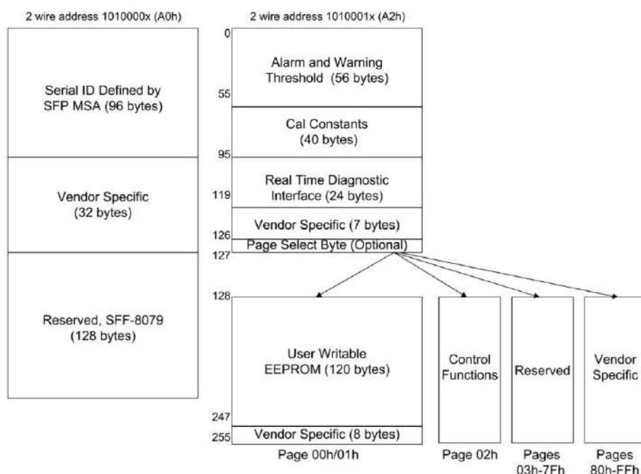
Figure4: Memory map
