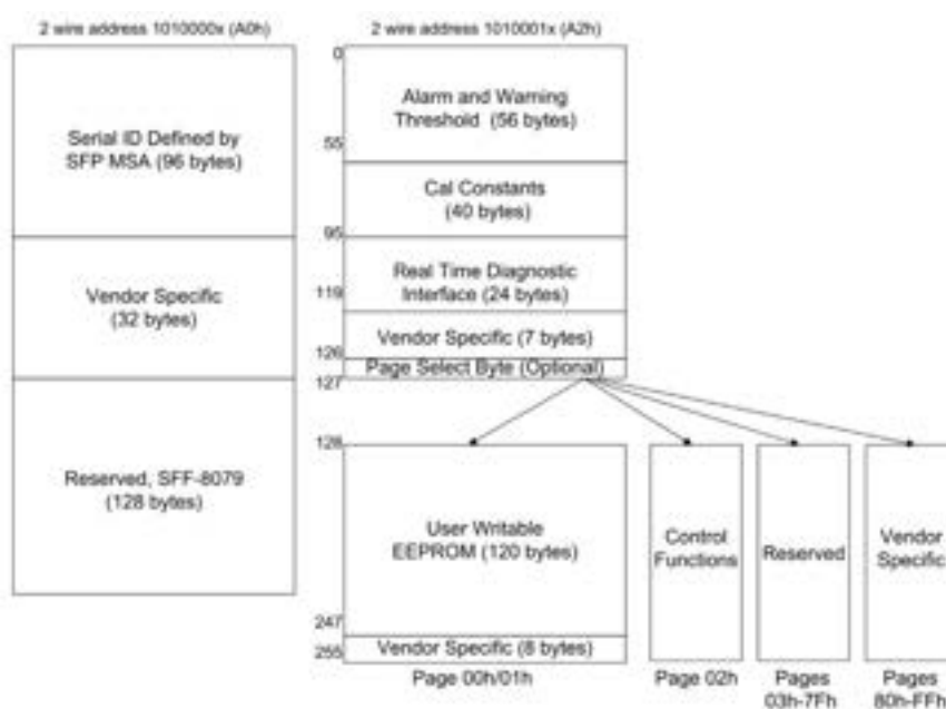
Figure4: Memory map
