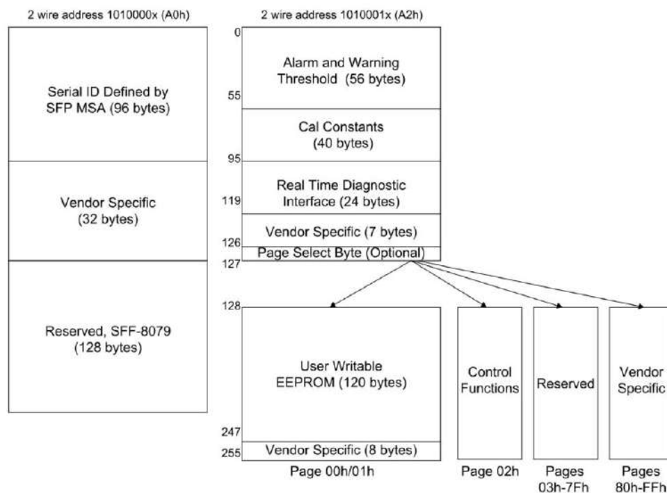
Figure4: Memory map
