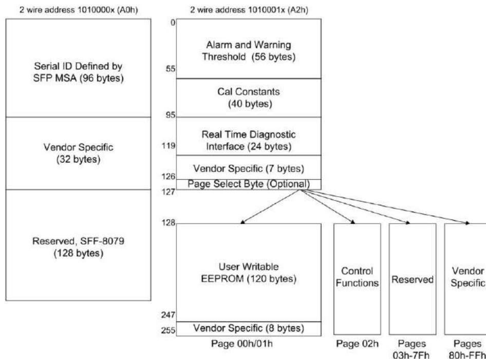
Figure4: Memory map
